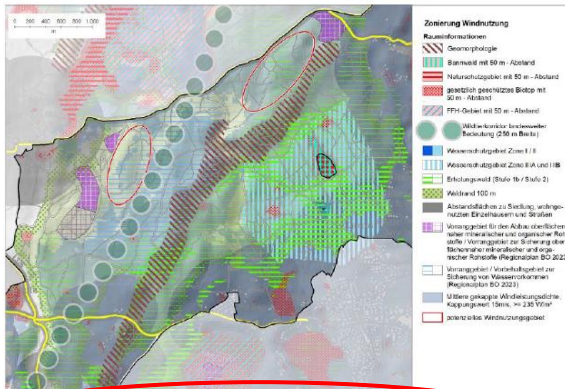
Abbildung 49: Zonierungsempfehlung Windenergie im Gebiet Waldburger Rücken
